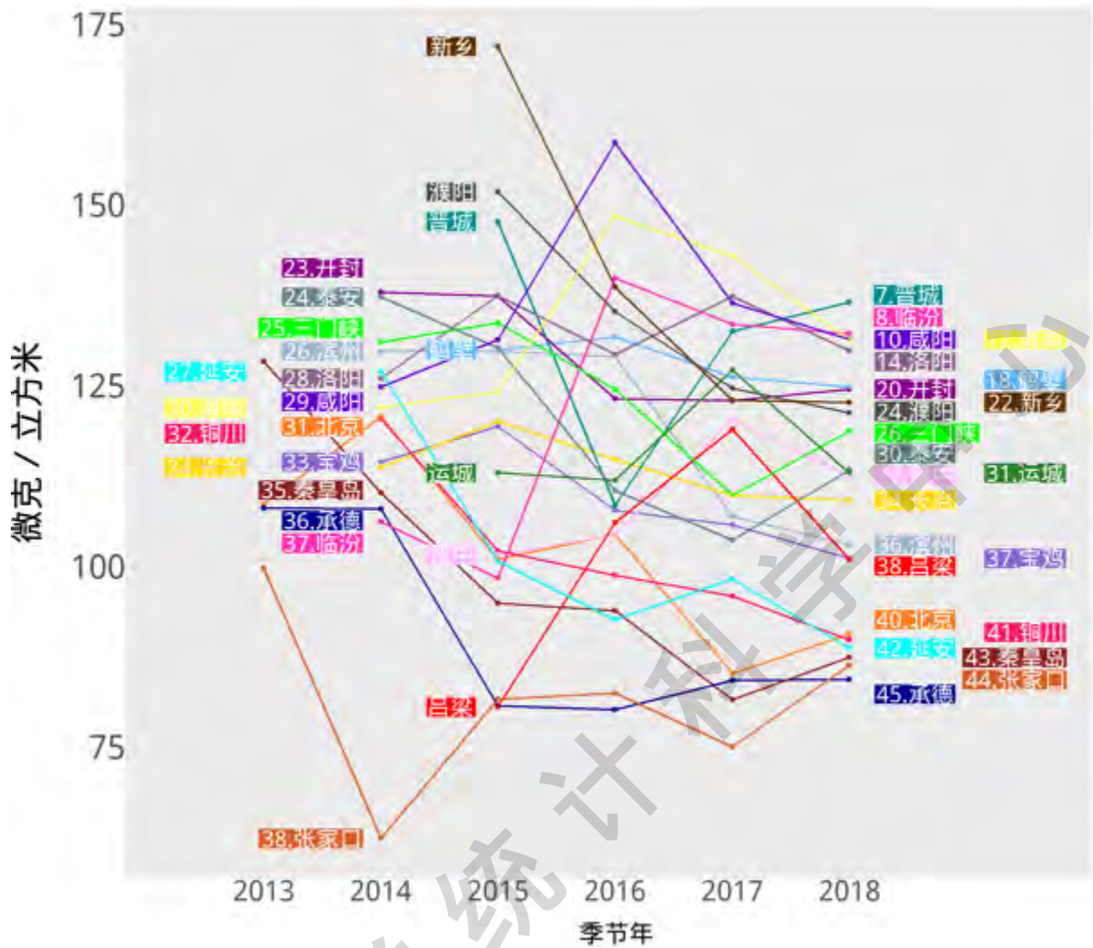
图 23：“2+43”城市后 23 名城市气象调整后 PM 10 季节年平均浓度(微克/立方米) 年际变化图 (新乡、濮阳、运城、鹤壁、晋城、晋中和吕梁因 2014 年部分季度数据缺失而给出 2015 年至 2018 年平均浓度)
