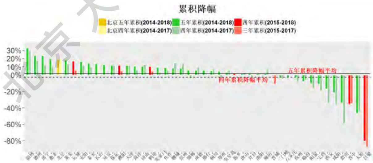
图 36：“2+43”城市气象调整后季节年二氧化氮过去五/四年（绿色）或过去四/三年（红色）累积降幅图 (红色表示因 2014 年部分季度数据缺失而计算的四/三年累积降幅)
