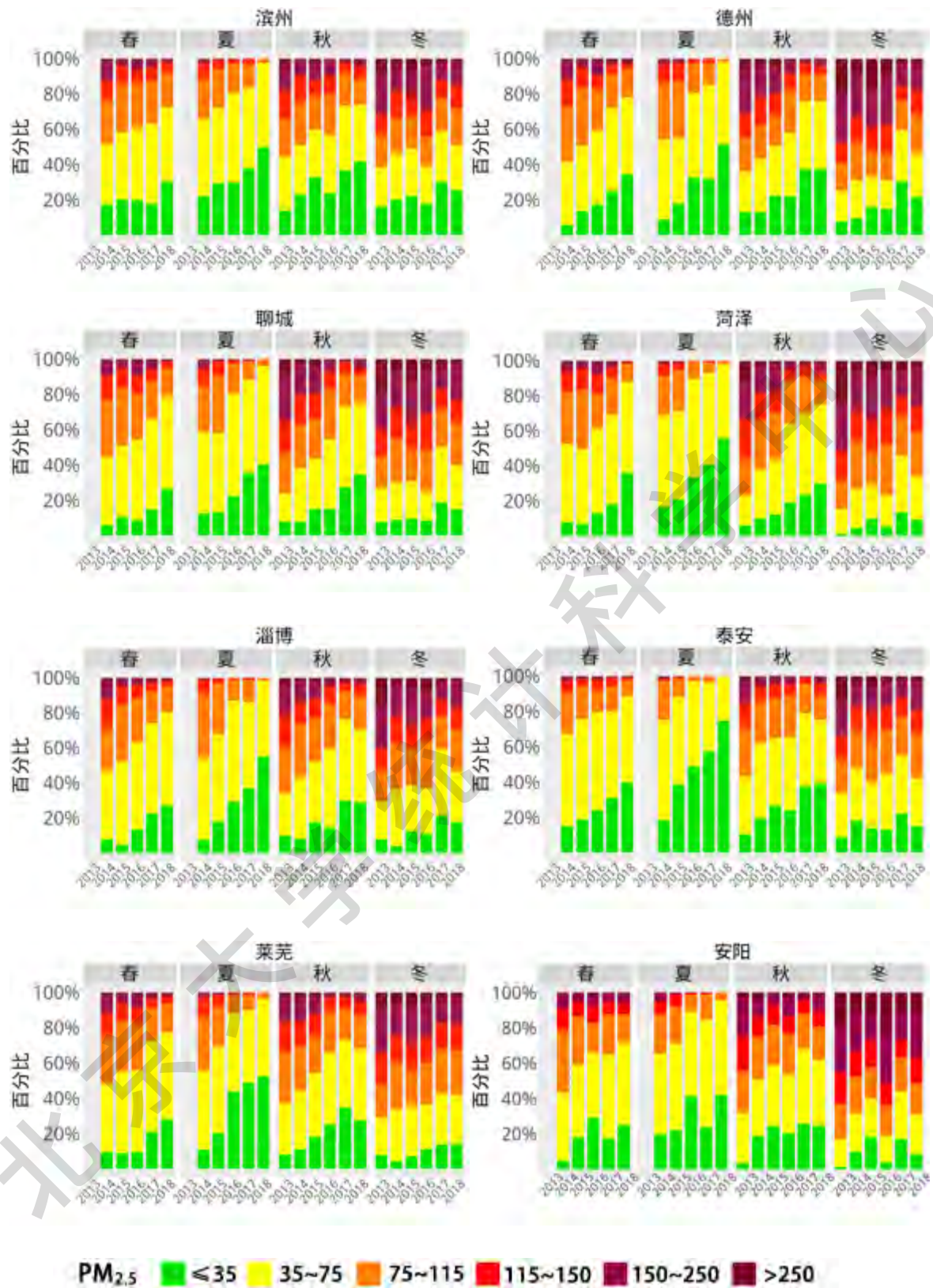
图 4：山东省 7 市和河南省 1 市 2013 年至 2018 年空气质量六个状态时间占比图
