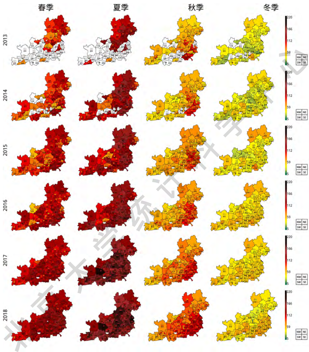
图 50：“2+43”城市 2013 年到 2018 年气象调整后 8 小时臭氧季节平均浓度(微克/立方米)地图 (白色代表数据少，无法得到可靠结果)
