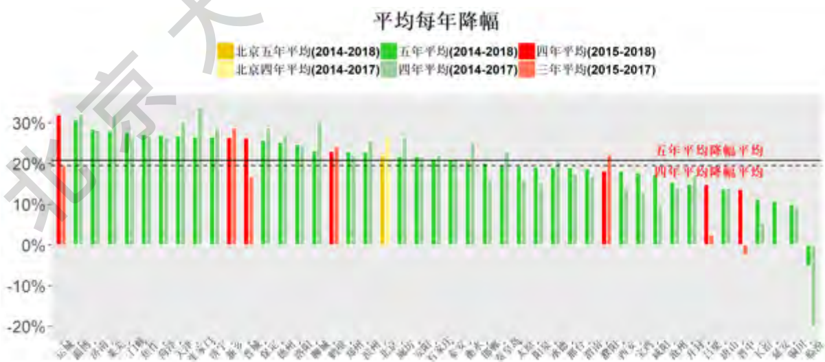
图 31：“2+43”城市气象调整后季节年二氧化硫过去五/四年（绿色）或过去四/三年（红色）平均降幅图 (红色表示因 2014 年部分季度数据缺失而计算的四/三年平均降幅)
