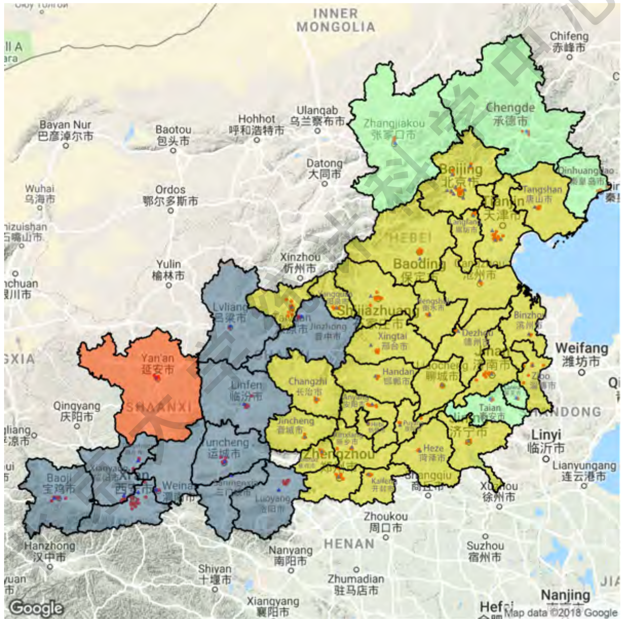
图 1：“2+43”城市区划及其站点分布（●代表空气质量监测站点，▲代表气象站点）
