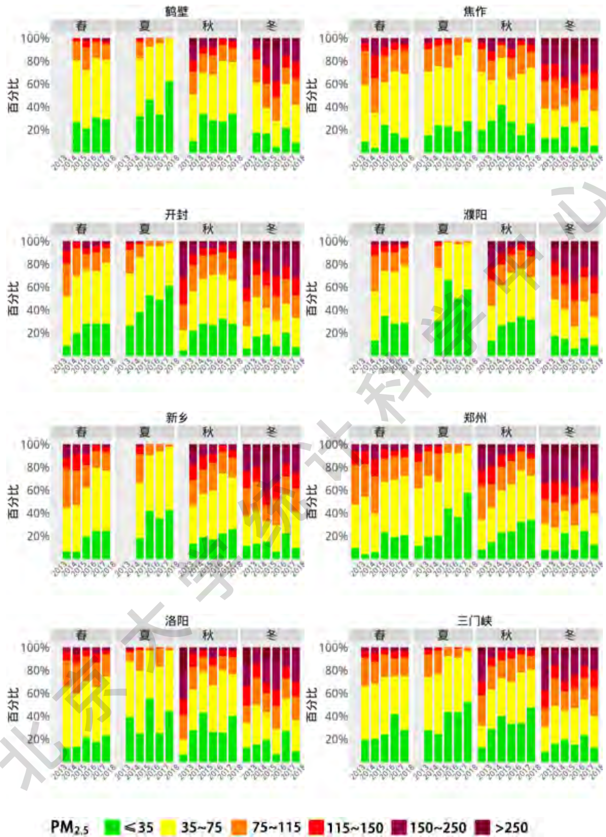
图 5：河南省 8 市 2013 年至 2018 年空气质量六个状态时间占比图
