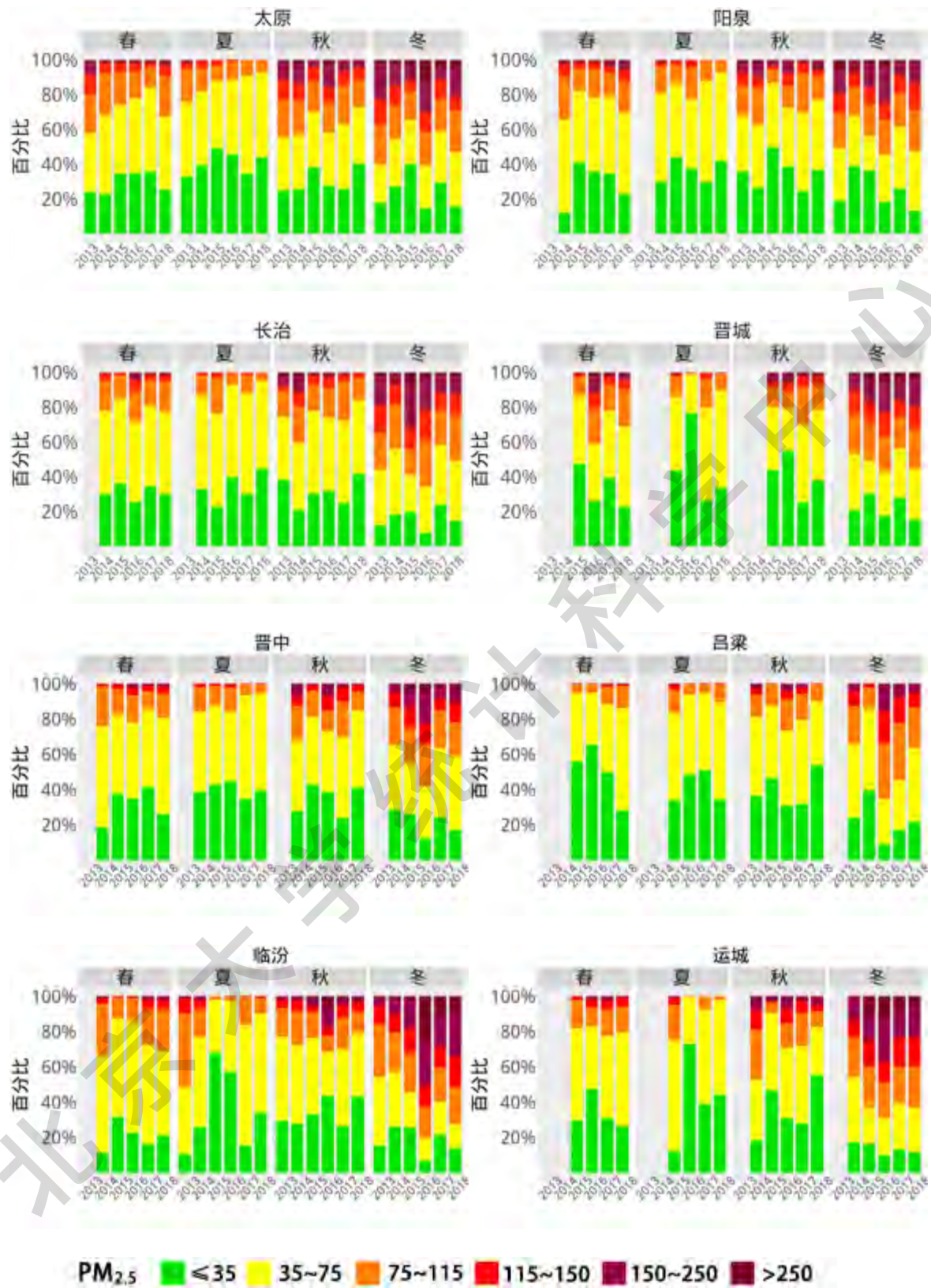
图6：山西省8市2013年至2018年空气质量六个状态时间占比图
