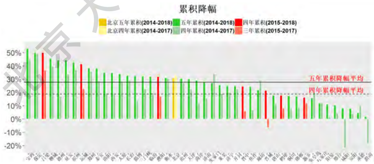
图 43：“2+43”城市气象调整后季节年一氧化碳过去五/四年（绿色）或过去四/三年（红色）累积降幅图 (红色表示因 2014 年部分季度数据缺失而计算的四/三年累积降幅)
