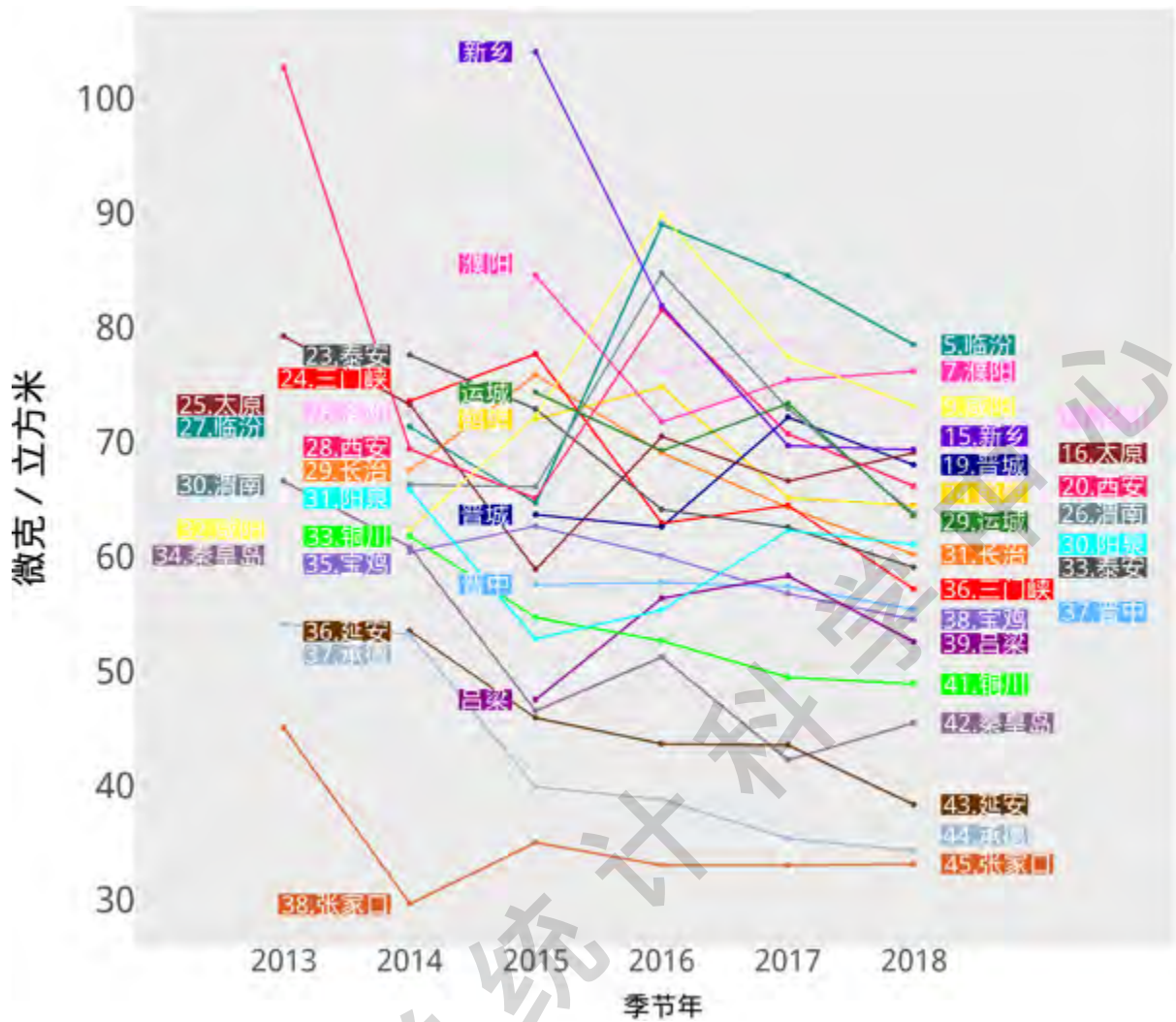
图 15：“2+43”城市后 23 名城市气象调整后 PM_{2.5} 季节年平均浓度(微克/立方米)年际变化图 (新乡、濮阳、运城、鹤壁、晋城、晋中和吕梁因 2014 年部分季度数据缺失而给出 2015 年至 2018 年平均浓度)
