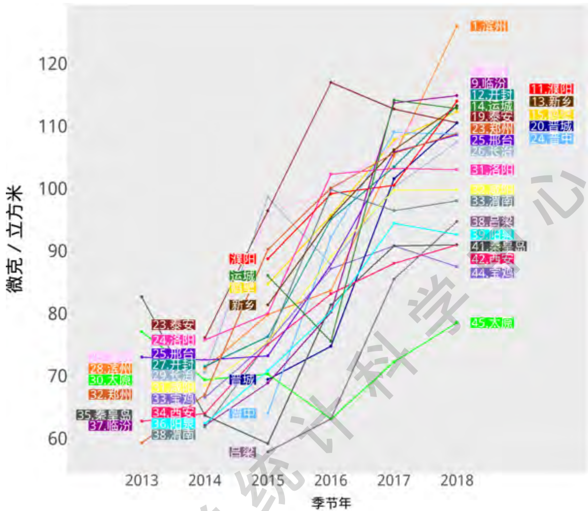
图 53：“2+43”城市气象调整后 23 名城市气象调整后 8 小时臭氧季节年平均浓度(微克/立方米) 年际变化 (新乡、濮阳、运城、鹤壁、晋城、晋中和吕梁因 2014 年部分季度数据缺失而给出 2015 年至 2018 年平均浓度)
