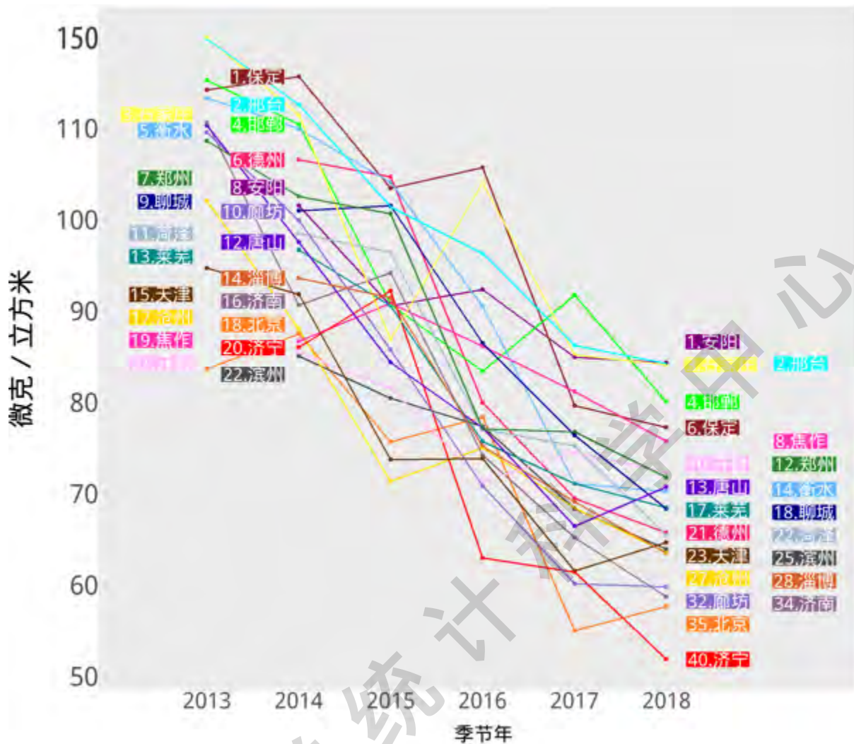
图 13：“2+43”城市前 22 名城市气象调整后 PM_{2.5} 季节年平均浓度(微克/立方米)年际变化图 (2014、2018 季节年的排名均以当年气象调整后的浓度为基准)
