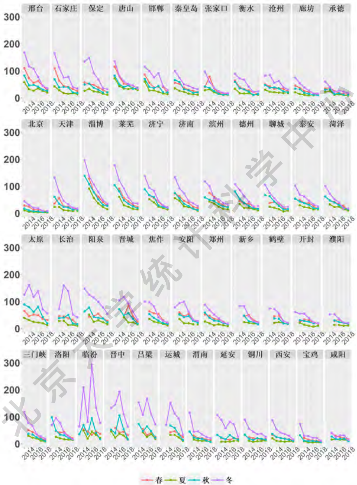
图 26：“2+43”城市气象调整后 2013 年至 2018 年二氧化硫季节平均浓度(微克/立方米)的变化序列图 图中实线（虚线）代表在 5% 统计学显著水平比上年有（无）显著增加或减少
